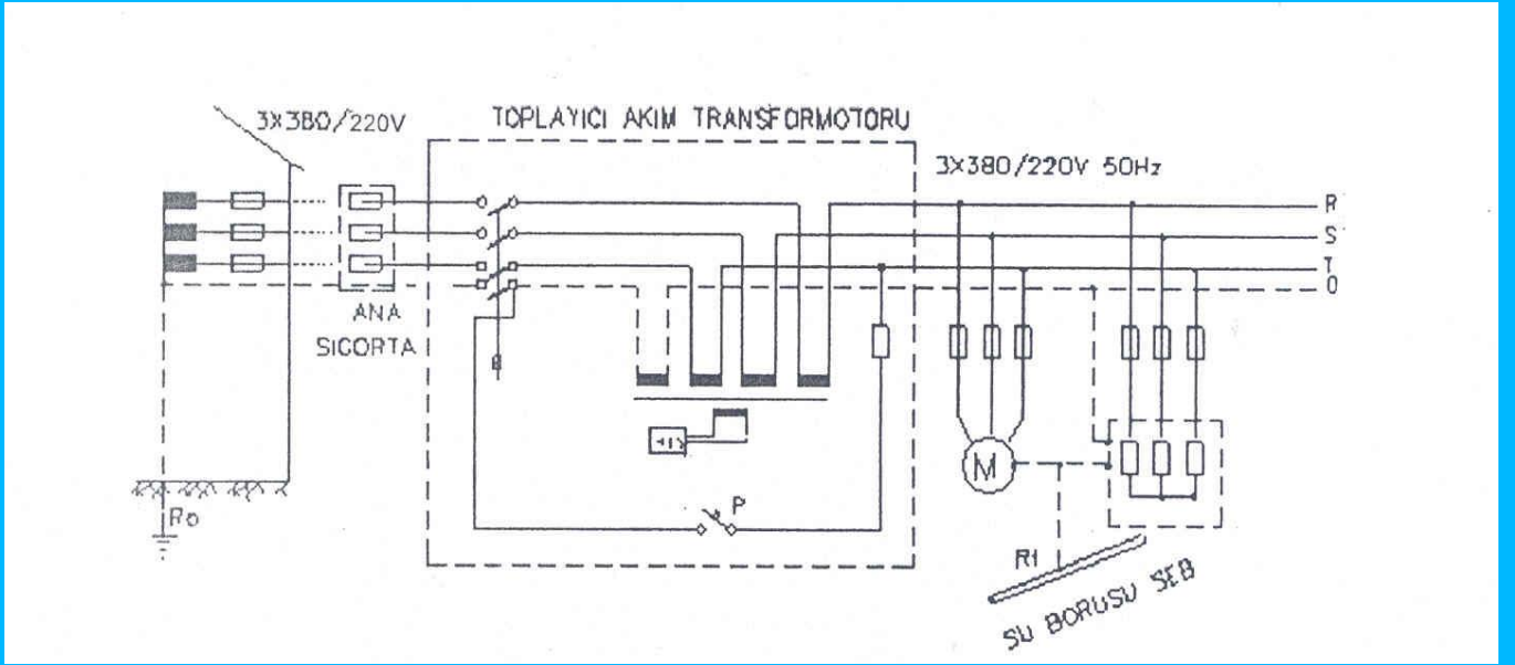
Şekil - 17 Hata akımı koruma bağlaması
