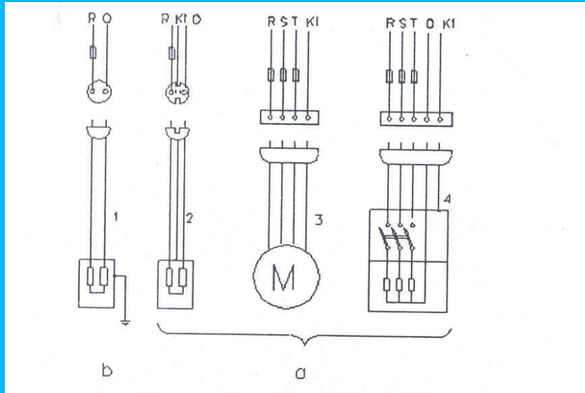
Şekil 8- Toprak teması akımının devresini su borusu şebekesi üzerinden kapadığı koruma topraklaması biçimleri
