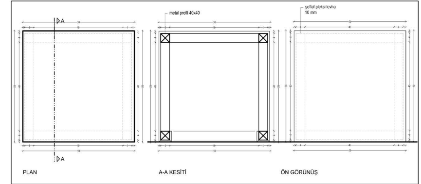
D1 - PANEL KATILIMCILARI OTURMA ÜNİTESİ DETAYI ÖLÇEK: 1/5
