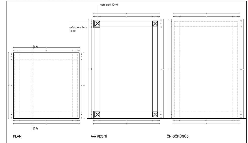
D2 - PANEL KATILIMCILARI SEHPA DETAYI ÖLÇEK: 1/5
