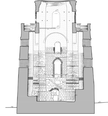
KESİT
