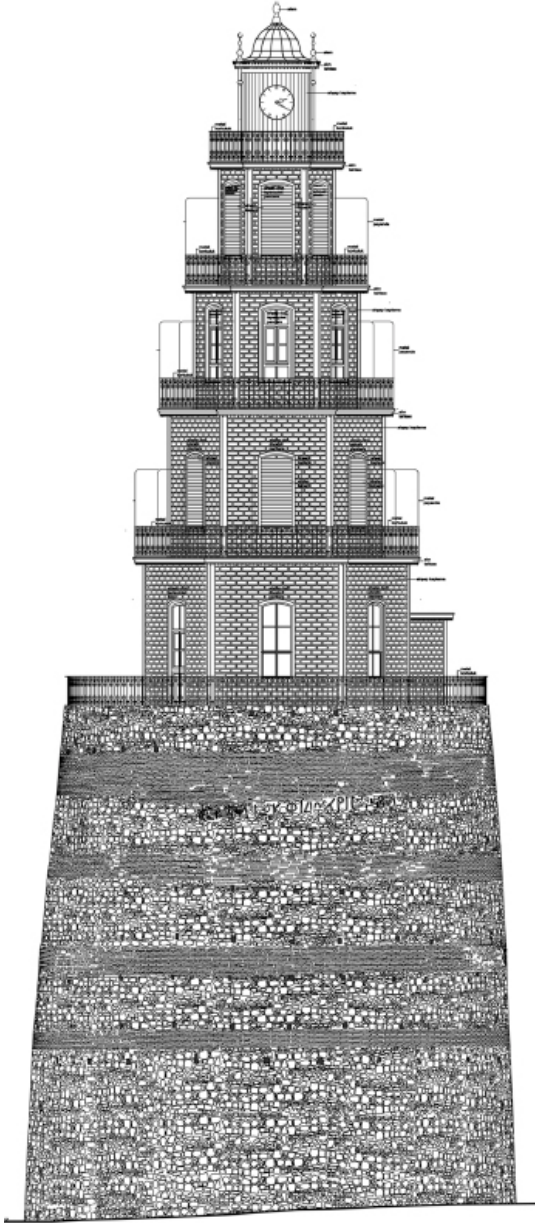
GÖRÜNÜŞ
