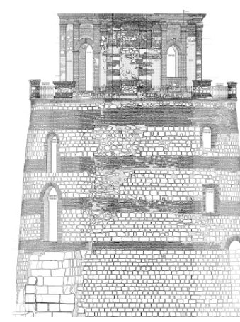
GÖRÜNÜŞ
