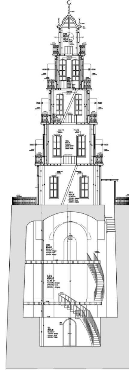
KESİT
